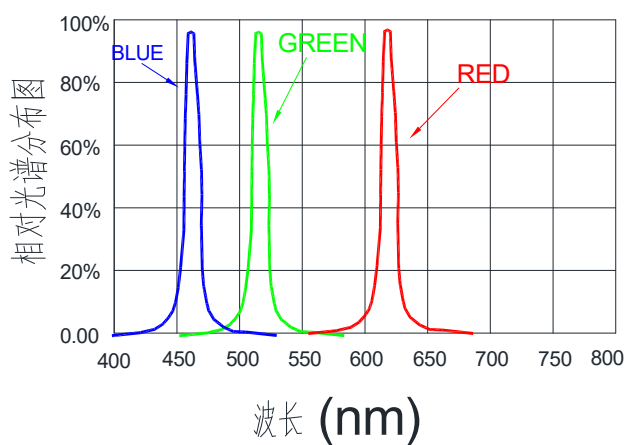
波长特性
